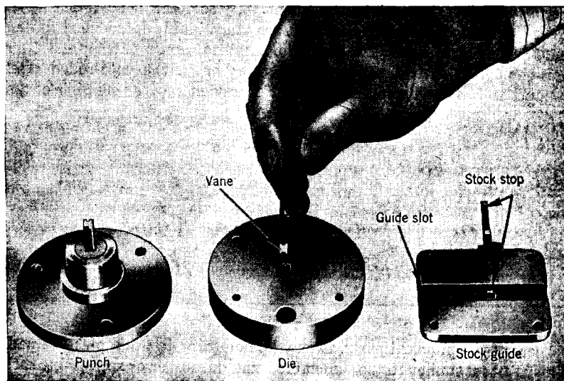
FIG. 17-1.—Vane-punching tools.
